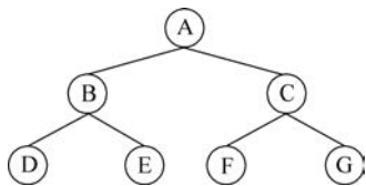
图 5.3 满二叉树
